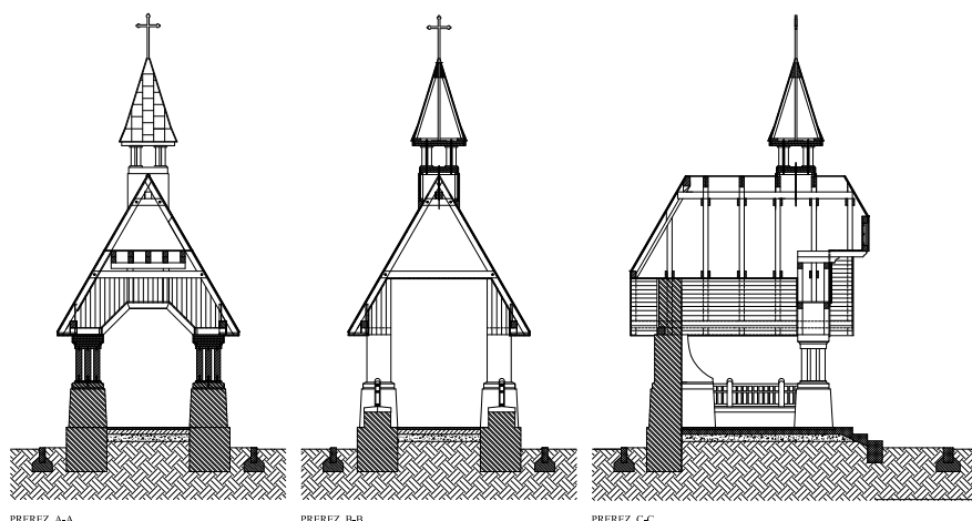
PREREZI A-A, B-B, C-C
